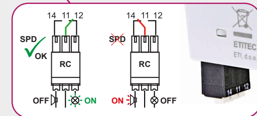
Styki sygnalizacji zdalnej (RC) uszkodzenia warystora.
