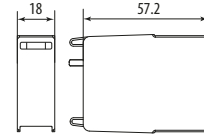
Moduł wymienny ETITEC ML T123 300/12,5
